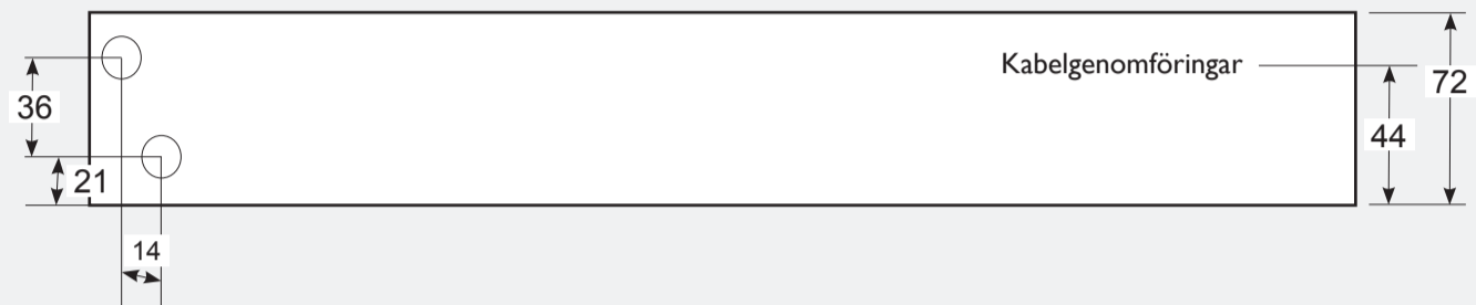
ÖVERSIKT OVANIFRÅN
