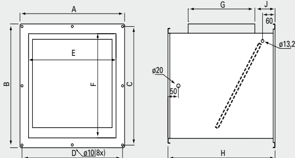
Blandningsskåp, SWBS
